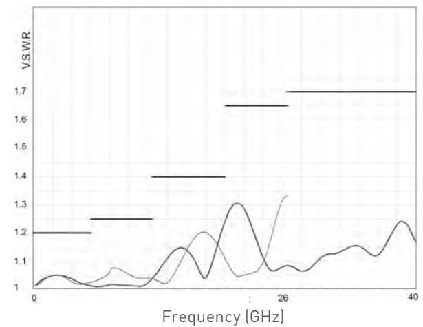
V.S.W.R.
