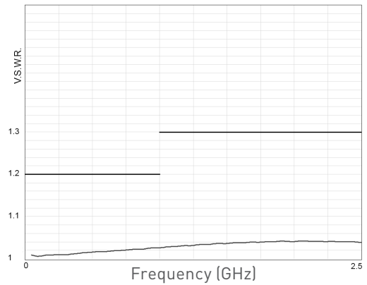
V.S.W.R.
