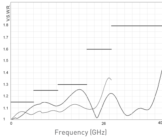
V.S.W.R.
