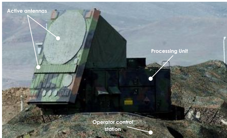
Fig. 1 : Phase array Radar (Patriot).
