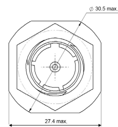
Size 9 MIL-DTL-38999 Connector
