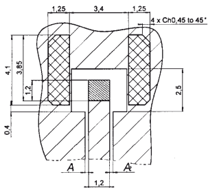
H3 Type Receptacle
